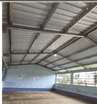
Foto 2:Módulo 1 y 2. Interior de la cubierta de techo y estructura metálica, instalada en los tres módulos de aulas.
